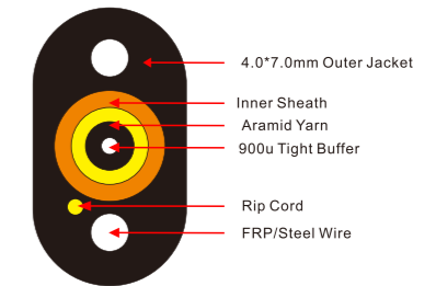
4.0*7.0mm
