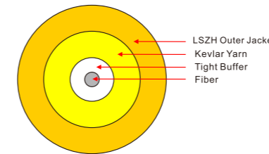
3.0mm
